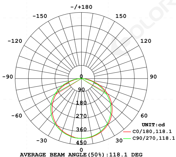
配光曲线图
